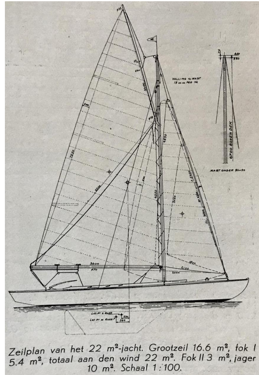
Tekening zonder kajuit in Waterkampioen van 3 mei 1935
